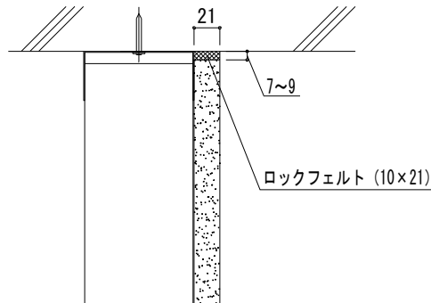
②床部 <ロックフェルト幅21mmなどの場合>
