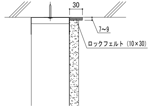
<ロックフェルト幅30mmの場合>
